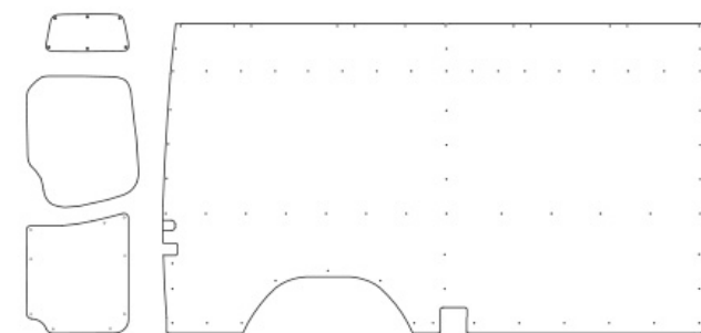
Version "2" - Heck/Front - C-/B-Säule
